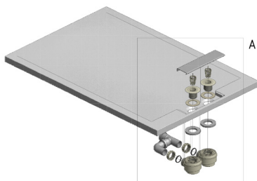
Double siphon (diamètre : 2 x 60 mm)
